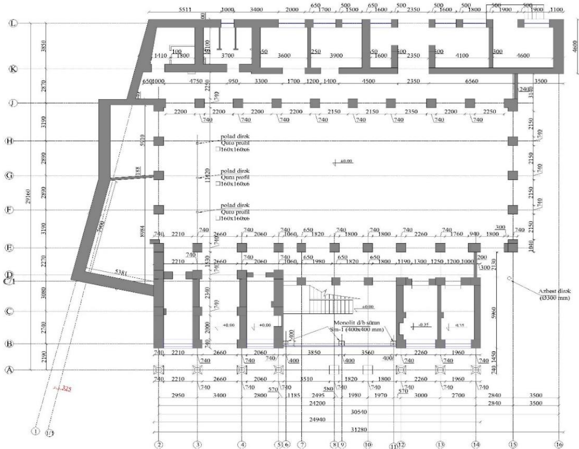
Şək. 6. Birinci mərtəbənin planı ( \pm 0.00 və -0.350 səviyyəsi)
