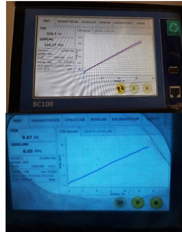
Şək. 4. Nümunələrin sınaqları (a-qaya daşı, b- qırmızı kərpic)
