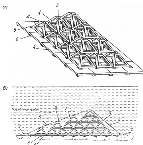
Рис. 8. Искусственный риф – подводный волнолом по патенту РФ №2314386:
