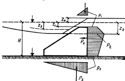
Рис. 4. Этюра волнового давления на подводный волнолом
