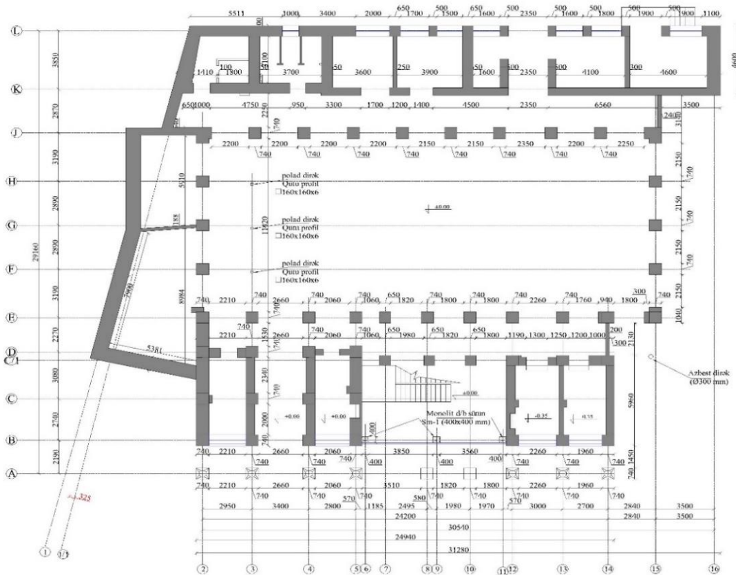
Şək. 6. Birinci mərtəbənin planı (±0.00 və -0.350 səviyyəsi)
