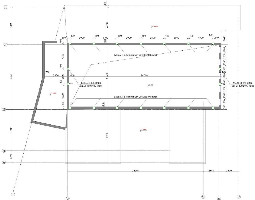
Şəkil 8. Binaının +7.60 səviyyəsində divar hörgüsünün planı
