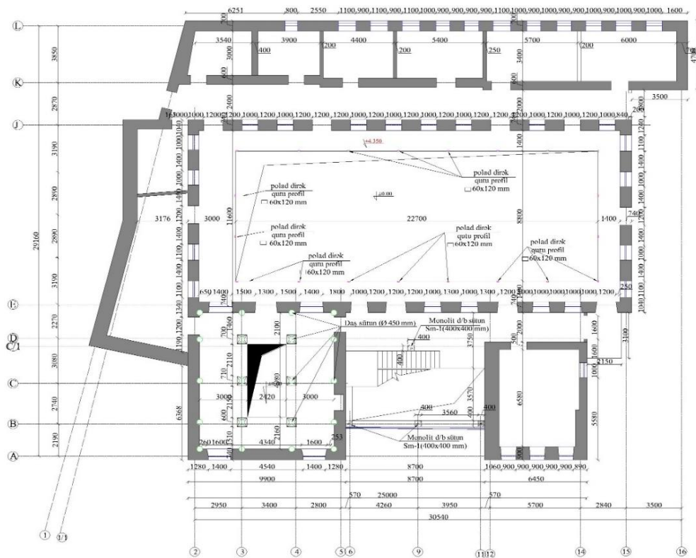
Şəkil 7. İkinci mərtəbənin planı (+4.350 səviyyəsi)
